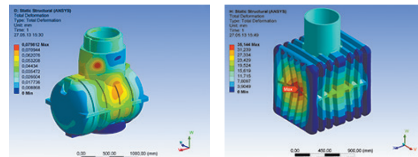
Деформация заполненного водой корпуса, при условии его заглубления на 1,7 м (по горловину)
